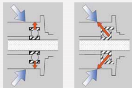
Průmyslové ložisko
