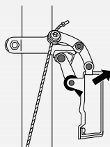
Přesmykač Down swing
